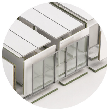
Schema connessioni e inserimento porte e finestre
